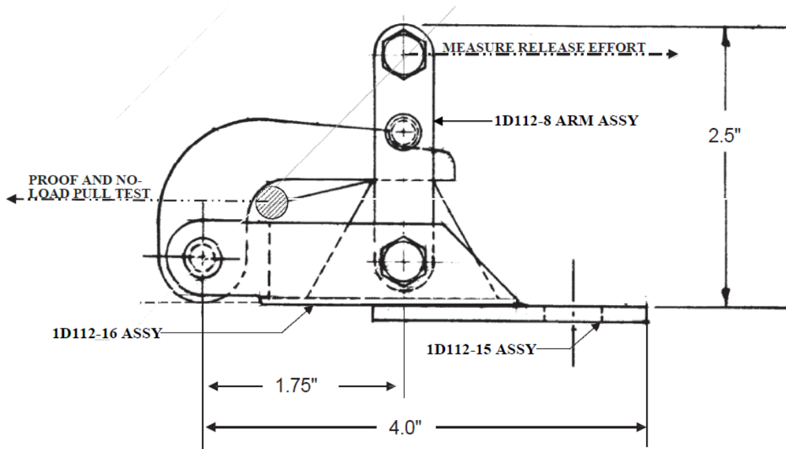
Figure 9-10. Schweizer Type Hitch
